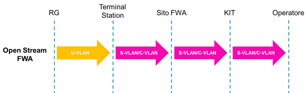
Figura 17 - Distribuzione VLAN per OpenStream FWA
