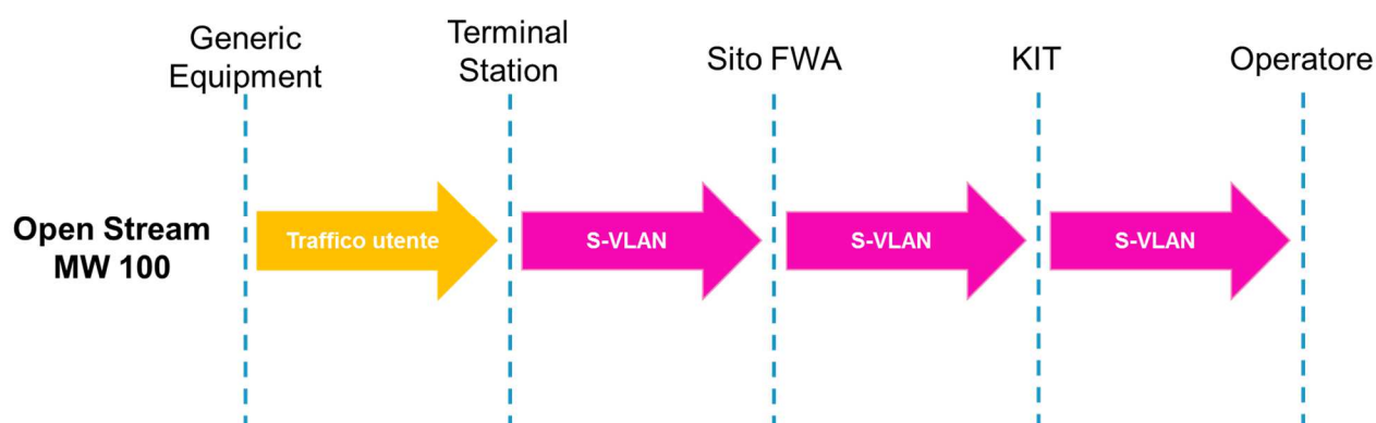
Figura 21 - Distribuzione VLAN per OpenStream MW100
