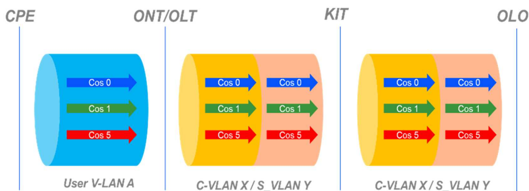
Figura 14 - Modello Multi CoS Double Tag
